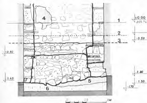
Сл. 8. — Изглед темеља зида апсиде ђаконикона: 1) ниво пода из 1906. год. (садашњи под); 2) ниво пода из XI века; 3) ниво пода из X века; 4) трагови најстаријег живописа (X в.); 5) касноантички слој; 6) здравица. — Fig. 8. — Vue de la fondation du mur de l'abside du diakonikon: 1) Niveau du sol de 1906 (sol actuel); 2) Niveau du sol du XI e s.; 3) Niveau du sol du X e s.; 4) Vestiges des plus anciennes fresques (X e s.); 5) Couche de la basse antiquité; 6) Sol vierge.
