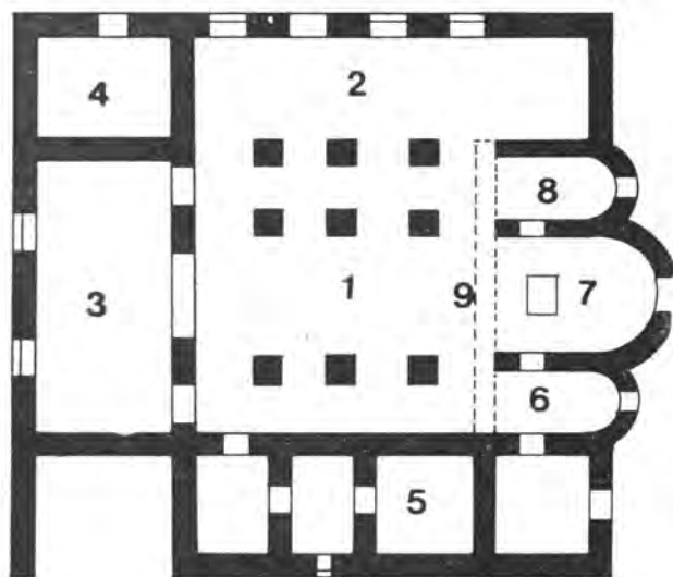
Сл. 2. — Основа цркве Св. Прокопија према М. Спиридоновићу-Пелеху; 1) средњи део храма; 2) туторско одељење; 3) притвор; 4) звонара; 5) гробница; 6) ђаконикон; 7) олтар; 8) проскомидија; 9) солеја. — Fig. 2. — Relevé de l'église Saint-Procopie d'après M. Spiridonović-Peleh: 1) Partie médiane du temple; 2) Pièce des tuteurs; 3) Pièce d'enfermement; 4) Clocher; 5) Tombeau; 6) Diakonikon; 7) Autel; 8) Proscomidie; 9) Soléa.
