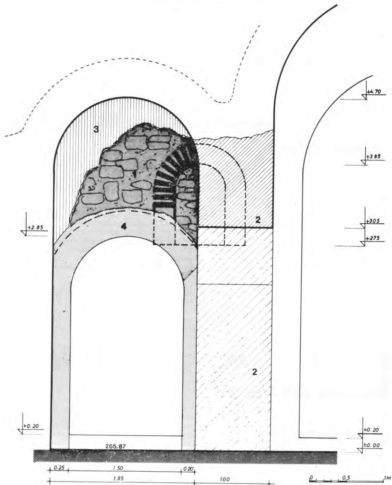
Сл. 19. — Попречни пресек кроз јужни брод цркве са погледом на западни зид наоса: 1) прва градитељска фаза (X век); 2) друга градитељска фаза (XI век); 3) трећа градитељска фаза (1734. год.); обнова цркве из 1906. год. — Fig. 19. — Section longitudinale de la nef sud de l'église avec vue du mur ouest du naos: 1) Première phase de construction (Xe s.); 2) Deuxième phase construction (XIe s.); 3) Troisième phase de construction (1734); 4) Rénovation de l'église en 1906.
