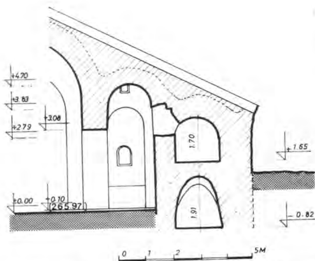
Сл. 22. — Попречни пресек кроз јужни брод цркве и гробницу св. Прокопија, према А. Радовићу и М. Медведеву. — Fig. 22. — Section longitudinale de la nef sud de l'église et du tombeau de saint Procope, d'après A. Radović et M. Medvedev.
