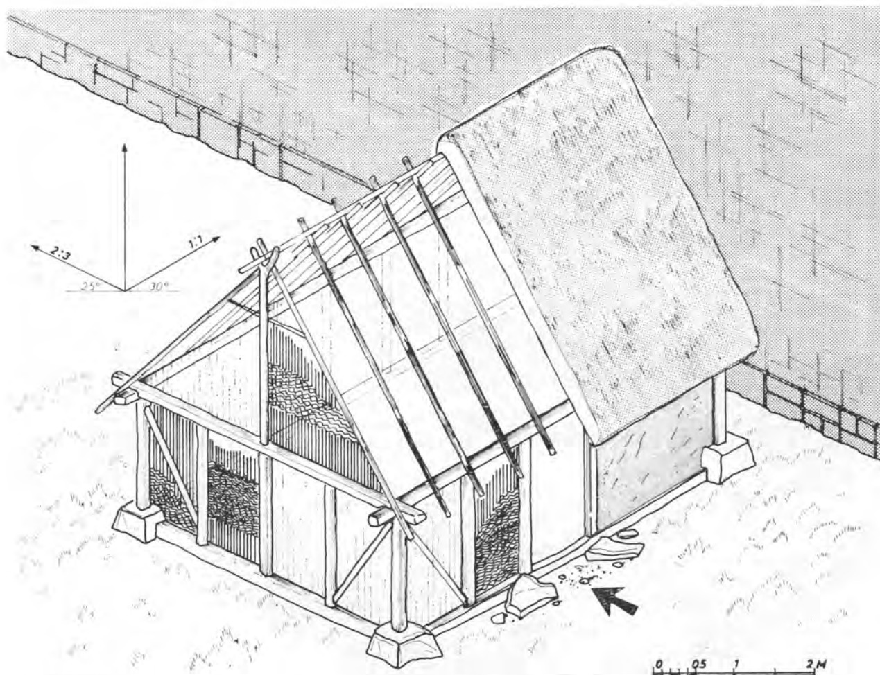
Сл. 18. — Реконструкција изгледа куће 4. — Fig. 18. — Reconstitution de l'aspect de la maison 4.
