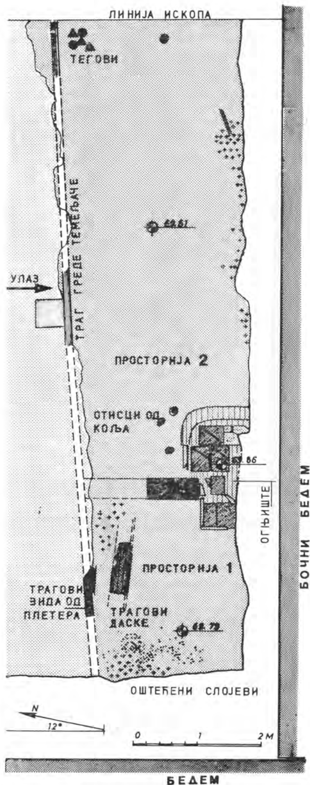
Сл. 13. — Основа куће 1. — Fig. 13. — Plan de la maison 1.
