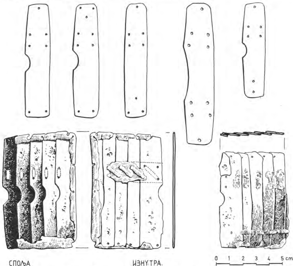
Сл. 23. — Типови плочица оклопа са остацима кожных трака (цртеж Н. Степановић). — Fig. 23. — Types of armor plates with remnants of leather straps (drawn by N. Stepanović).
