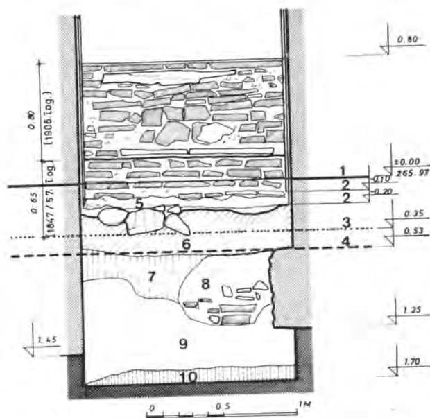
Сл. 23. — Пресек кроз апсиду ђаконикона: 1) ниво пода из 1906. год. (садашњи под); 2) ниво пода из средине XIX века; 3) ниво пода из XI века; 4) ниво пода из X века; 5) трагови малтера бојени секо техником; 6) слој из средине XIX века; 7) средњевековни слој; 8) позносредњевековни укуп; 9) касноантички слој; 10) здравица. — Fig. 23. — Section longitudinale de l'abside du diakonikon: 1) Niveau du sol de 1906 (sol actuel); 2) Niveau du sol du milieu du XIX e s.; 3) Niveau du sol du XI e s.; 4) Niveau du sol du X e s.; 5) Traces de mortier peint en technique sèche; 6) Couche du milieu du XIX e s.; 7) Couche médiévale; 8) Fosse de basse époque médiévale; 9) Couche de la basse antiquité; 10) Sol vierge.
