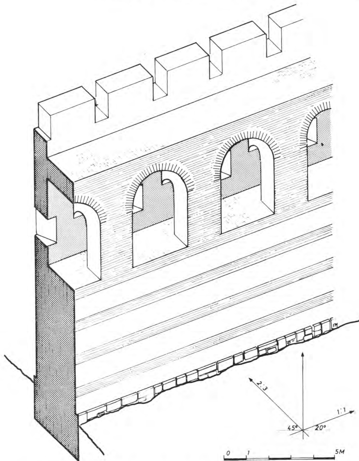
Сл. 5. — Реконструкција унутрашњег изгледа једног дела бедема. — Fig. 5. — Reconstitution de l'intérieur d'une partie de rempart.
