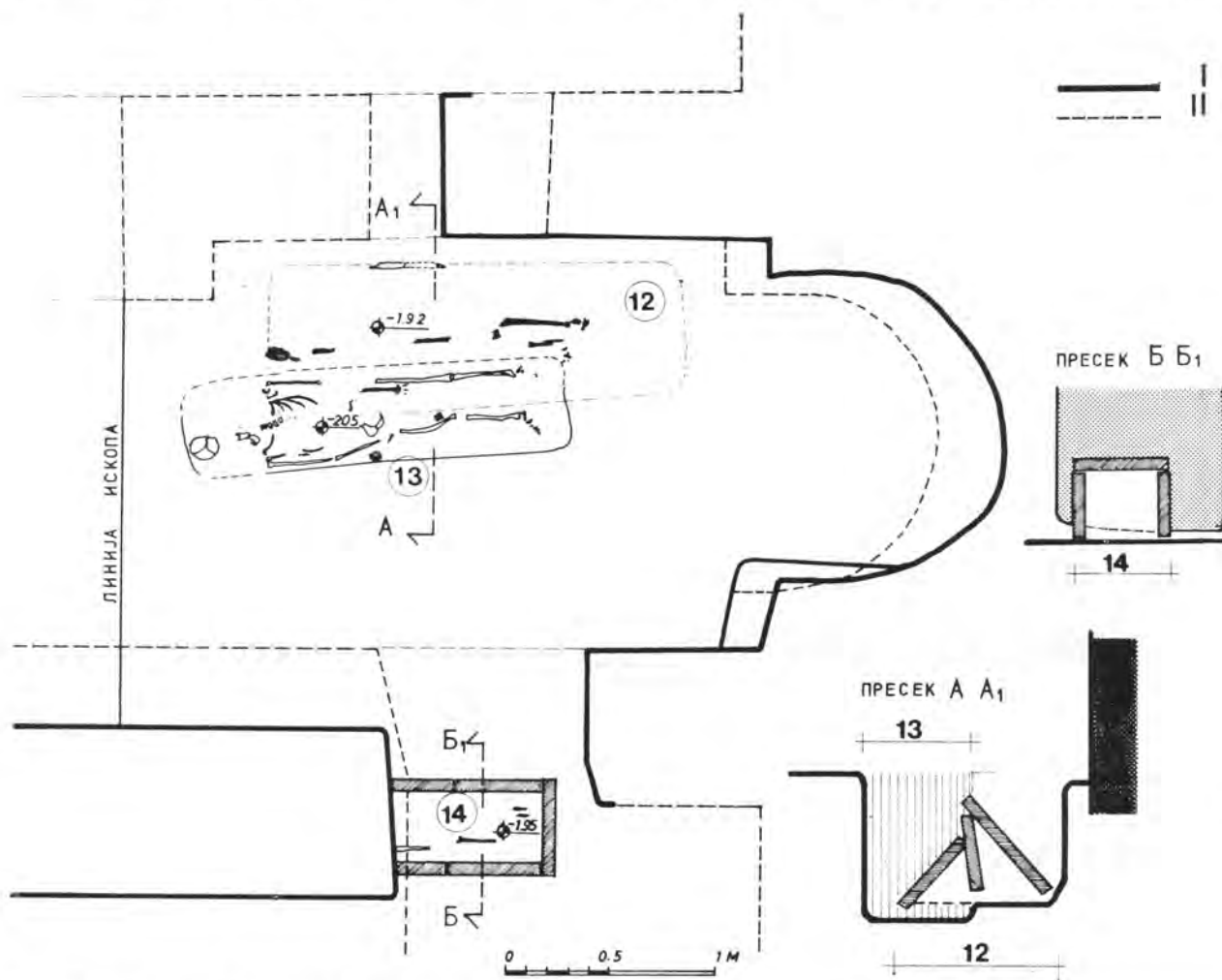
Сл. 25. — Старији хоризонт сахрањивања, гробови 12—14. — Fig. 25. — Horizon ancien d'ensevelissement, tombes 12—14.
