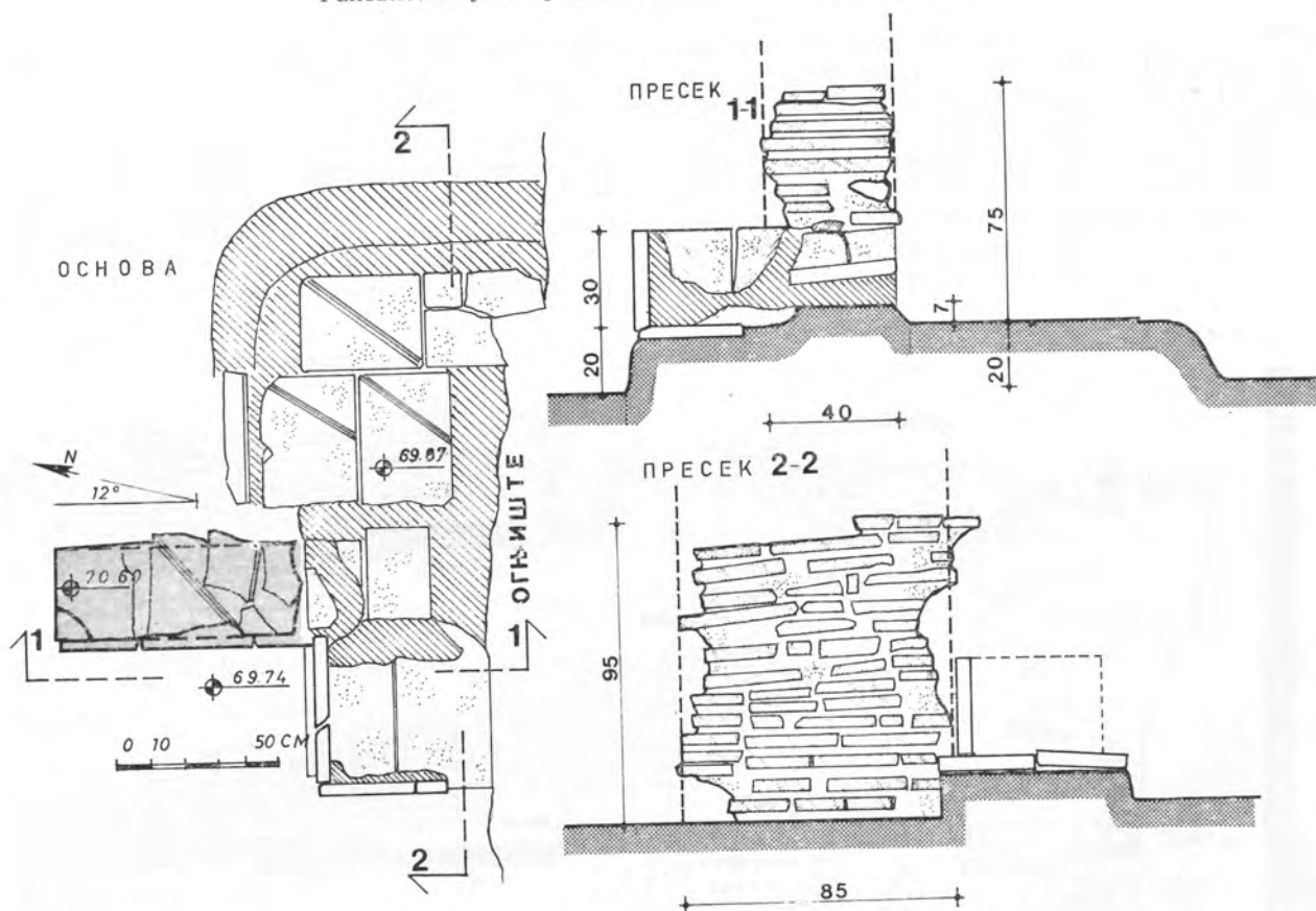
Сл. 14. — Детаљ преградног зида и огњишта у кући 1. — Fig. 14. — Détails de la cloison et du foyer dans la maison 1.
