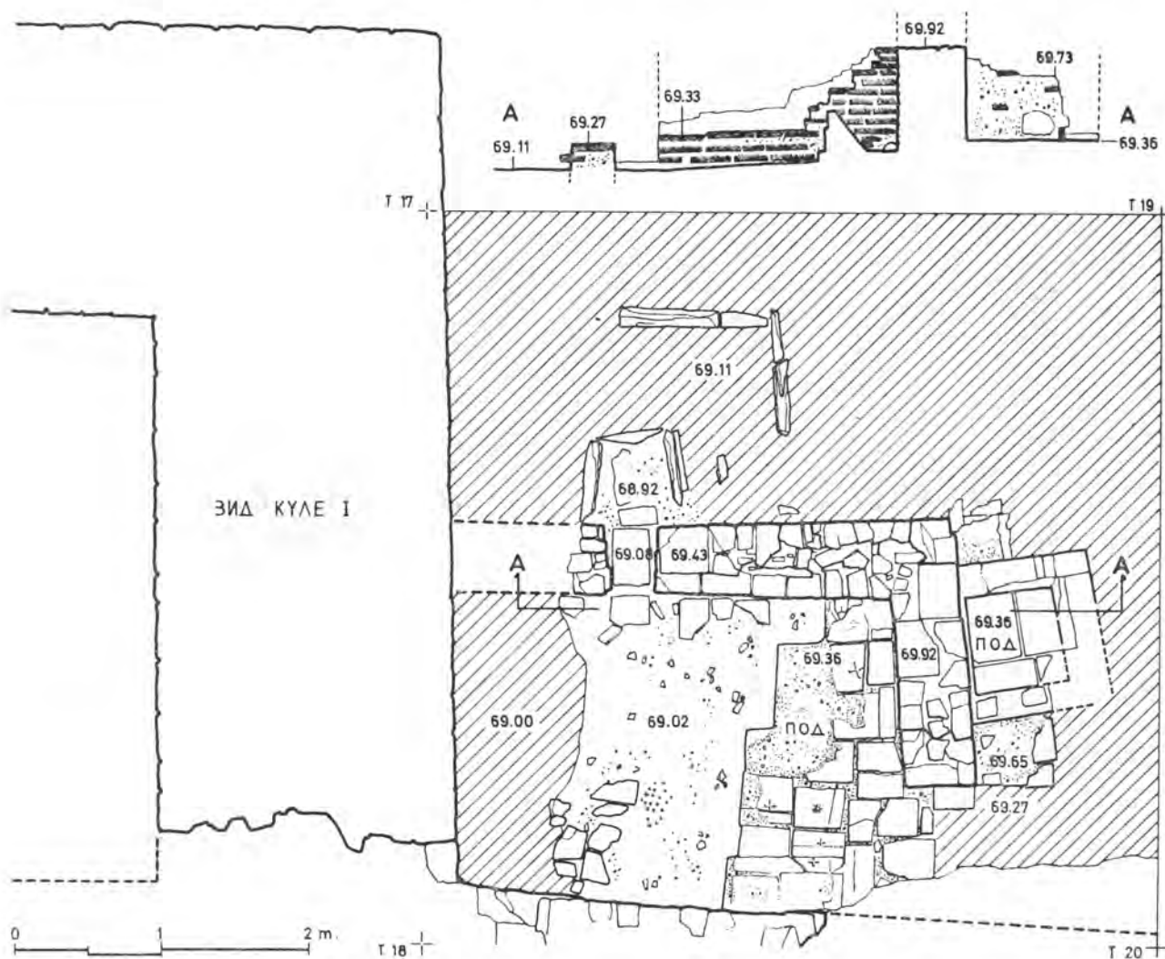
Сл. 11. — Објект уз кулу I, основа и пресек (цртеж Г. Милошевић). — Fig. 11. — Building along the Tower I, foundation and cross-section (drawn by G. Milošević).
