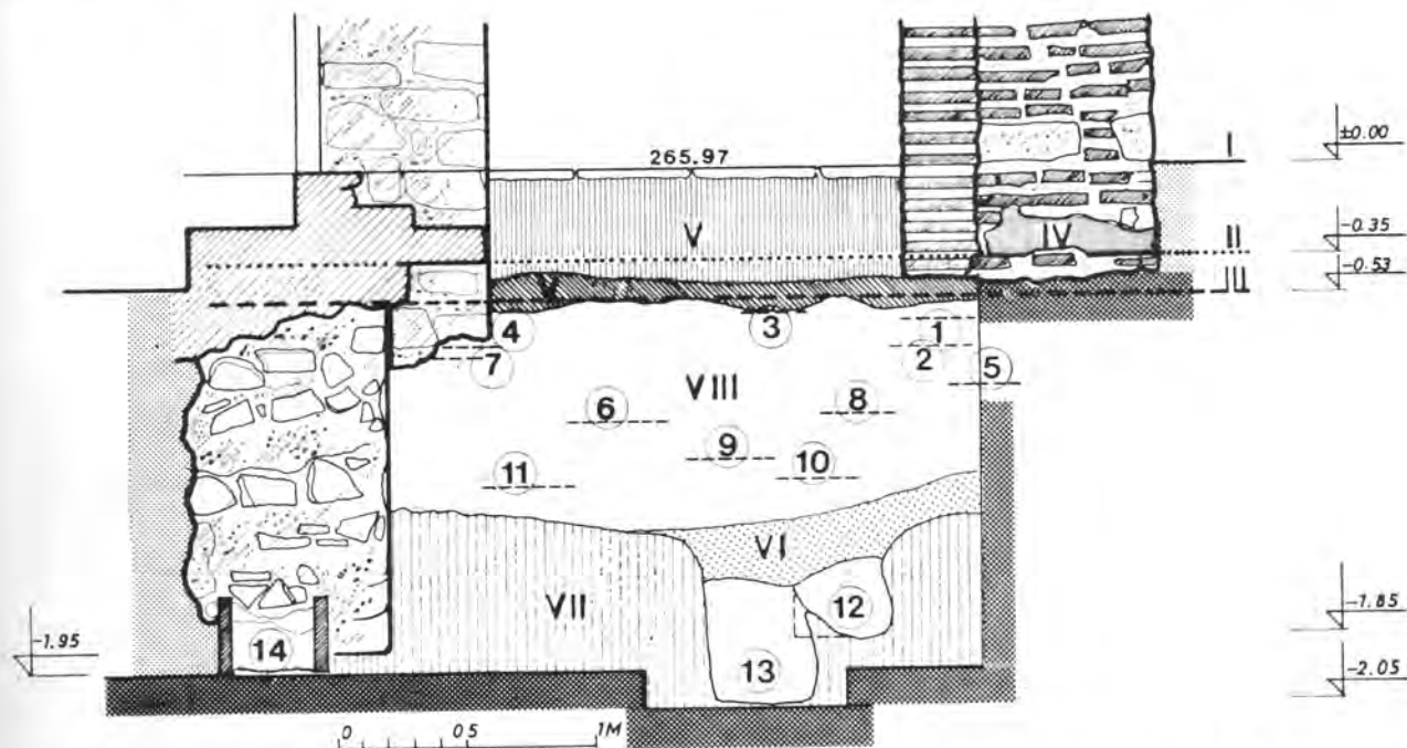
Сл. 24. — Вертикална стратиграфија и положај гробова у ђаконикону: I) ниво пода из 1906. год. (садашњи под); II) ниво пода из XI века; III) ниво пода из X века; IV) слој живописа из XI века; V) подлога за под из 1906. год.; VI) касноантички слој; VII) здравица; VIII) средњовековни слој, ниво уклањања гробова; 1—11) средњовековни гробови; 12—14) касноантички гробови. — Fig. 24. — Stratigraphie verticale et disposition des tombes dans le diakonikon: I) Niveau du sol de 1906 (sol actuel); II) Niveau du sol du XI e s.; III) Niveau du sol du X e s.; IV) Couche de fresques du XI e s.; V) Semelle du sol de 1906; VI) Couche de la basse antiquité; VII) Sol vierge; VIII) Couche médiévale, niveau des tombes; 1—11) Tombes médiévales; 12—14) Tombes de la basse antiquité.
