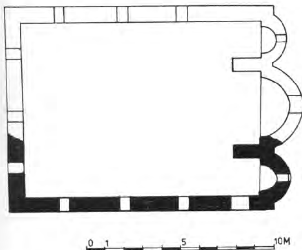
Сл. 20. — Основа цркве, прва градитељска фаза (X век). — Fig. 20. — Relevé de l'église, première phase de construction (X e s.).
