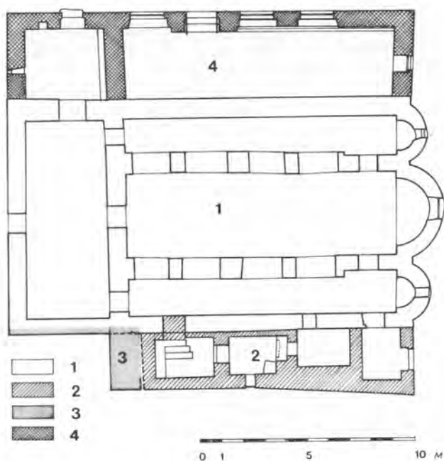
Сл. 16. — Основа цркве Св. Прокопија са претпостављеним градитељским фазама: 1) тробродна базилика; 2) гробница св. Прокопија; 3) преправка југозападнoг угла цркве; 4) турско одељење и крстионица (звонара). — Fig. 16. — Relevé de l'église Saint-Procope avec phases de construction probables: 1) Basilique à trois neufs; 2) Tombeau saint Procope; 3) Remaniement de l'angle sud-ouest de l'église; 4) La pièce des tuteurs et le baptistère (clocher).
