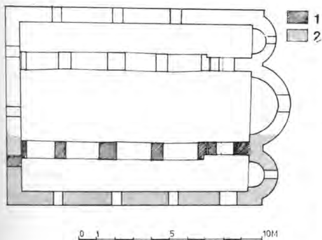
Сл. 21. — Основа тробродне базилике из XI века: 1) прва градитељска фаза; 2) друга градитељска фаза. — Fig. 21. — Relevé de la basilique à trois nefs du XI e s.: 1) Première phase de construction; 2) Deuxième phase de construction.
