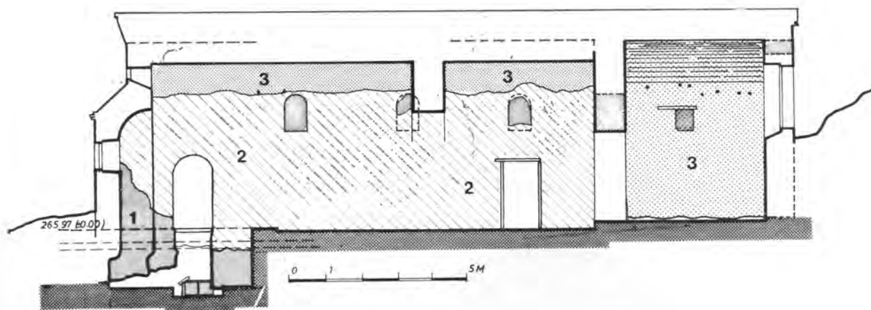
Сл. 18 — Подужни пресек кроз јужни брод цркве са погледом на јужни зид: 1 и 2) прва градитељска фаза (X век); 3) трећа градитељска фаза (1734. год.). — Fig. 18. — Section longitudinale de la nef sud avec vue du mur ouest du naos: 1 et 2) Première phase de construction (X e s.); 3) Troisième phase de construction (1734).
