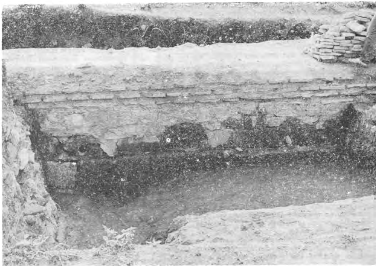
Сл. 3. — Спољно лице бедема на Светињи, детаљ у квадрату XXXVIII (спимио М. Поповић). — Fig. 3. — Outside view of the Svetinja rampart, detail in square XXXVIII (photographed by M. Popović).
