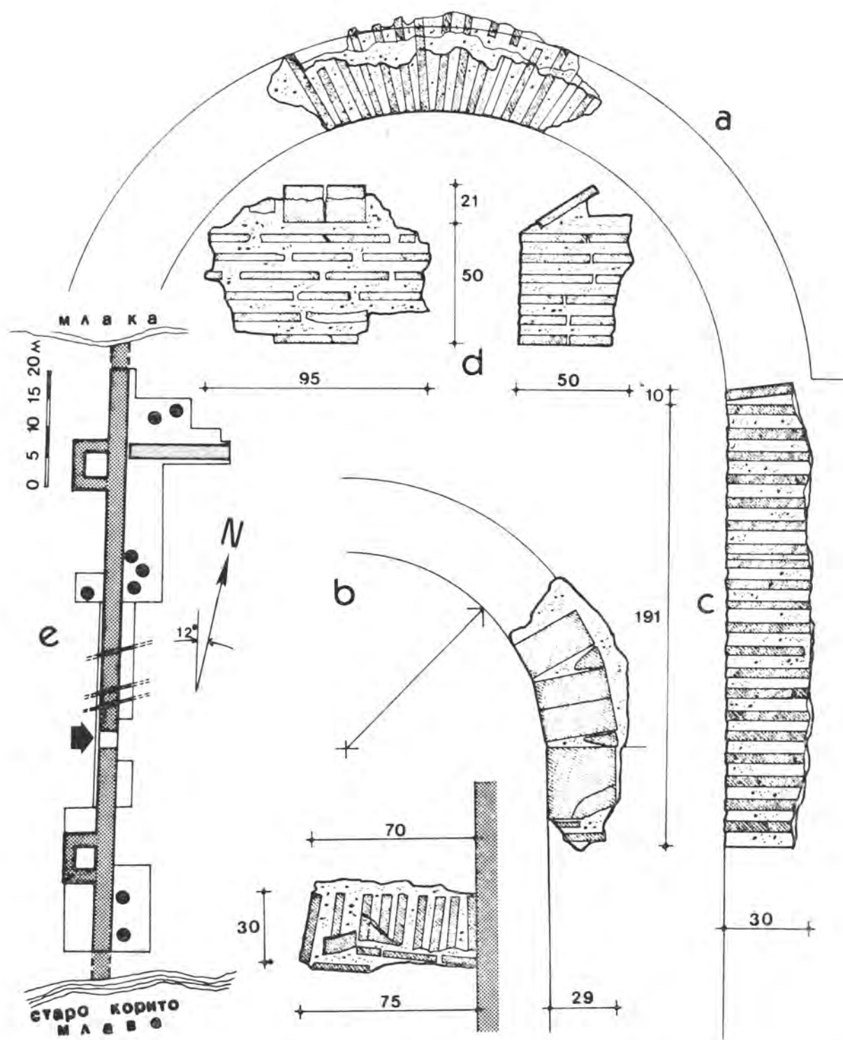
Сл. 1. — Детаљи урушених сводних конструкција бедема. — Fig. 1. — Détails des constructions voûtées du rempart en ruines.
