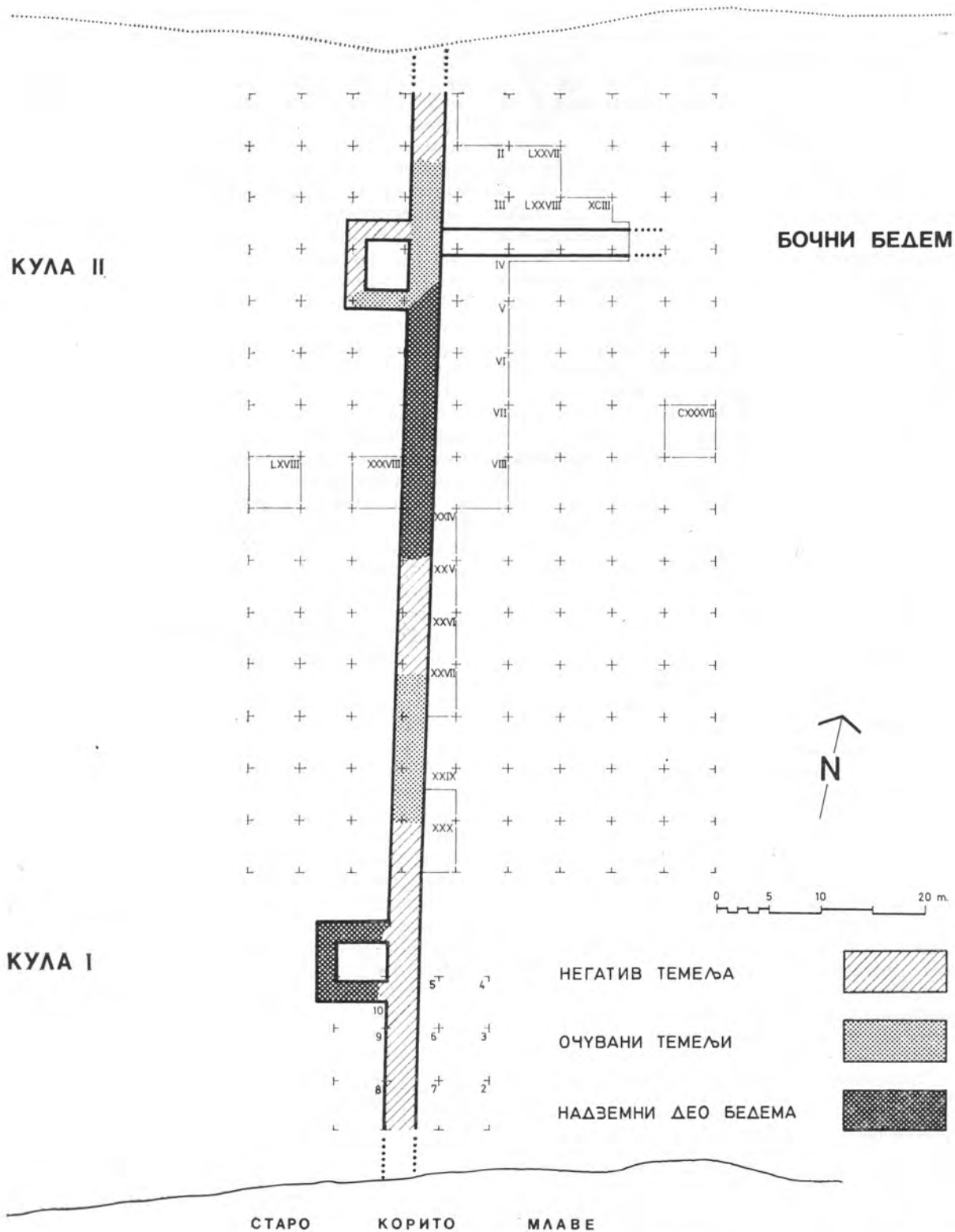
Сл. 2. — Ситуациони план локалитета на Светињи са основом рановизантијског бедема. — Fig. 2. — Layout of the Svetinja site with the foundations of the Early Byzantine rampart.
