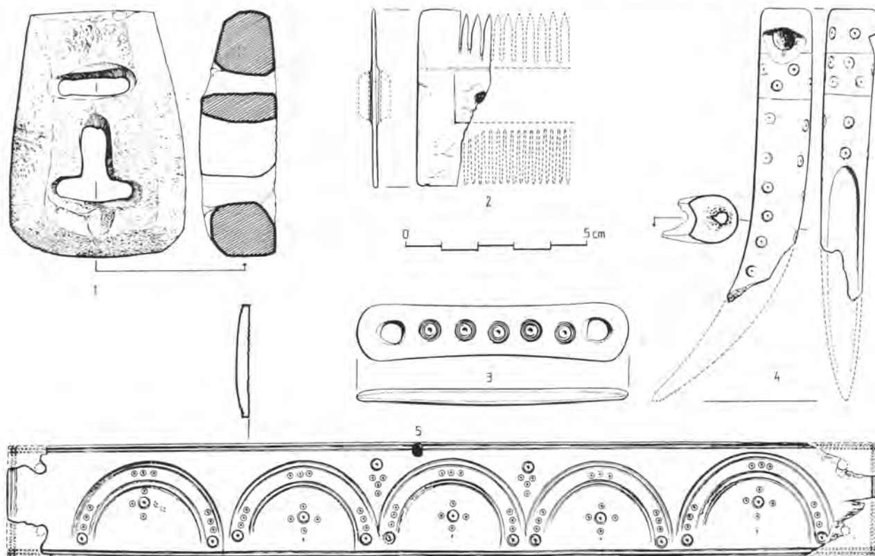
Сл. 20. — Коштани предмети из рановизантијских слојева на Светињи (цртеж Н. Степановић). — Fig. 20. — Bone artifacts from the Svetinja Early Byzantine layers (drawn by N. Stepanović).
