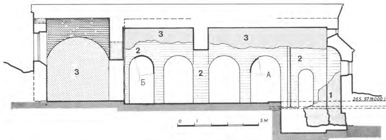
Сл. 17. — Подужни пресек кроз јужни брод цркве са погледом на северни зид: 1) прва градитељска фаза (X век); 2) друга градитељска фаза (XI век); 3) трећа градитељска фаза (1734. год.): А) Св. ратник, фреска из X в.; Б) Св. Пахомије, херувим, фреске из XIV в. — Fig. 17. — Section longitudinale de la nef sud avec vue du mur nord: 1) Première phase de construction (X e s.); 2) Deuxième phase de construction (XI e s.); 3) Troisième phase de construction (1734); А) Saint militaire, fresque du XI e s.; Б) Saint Pacôme, chérubin, fresques du XIV e s.
