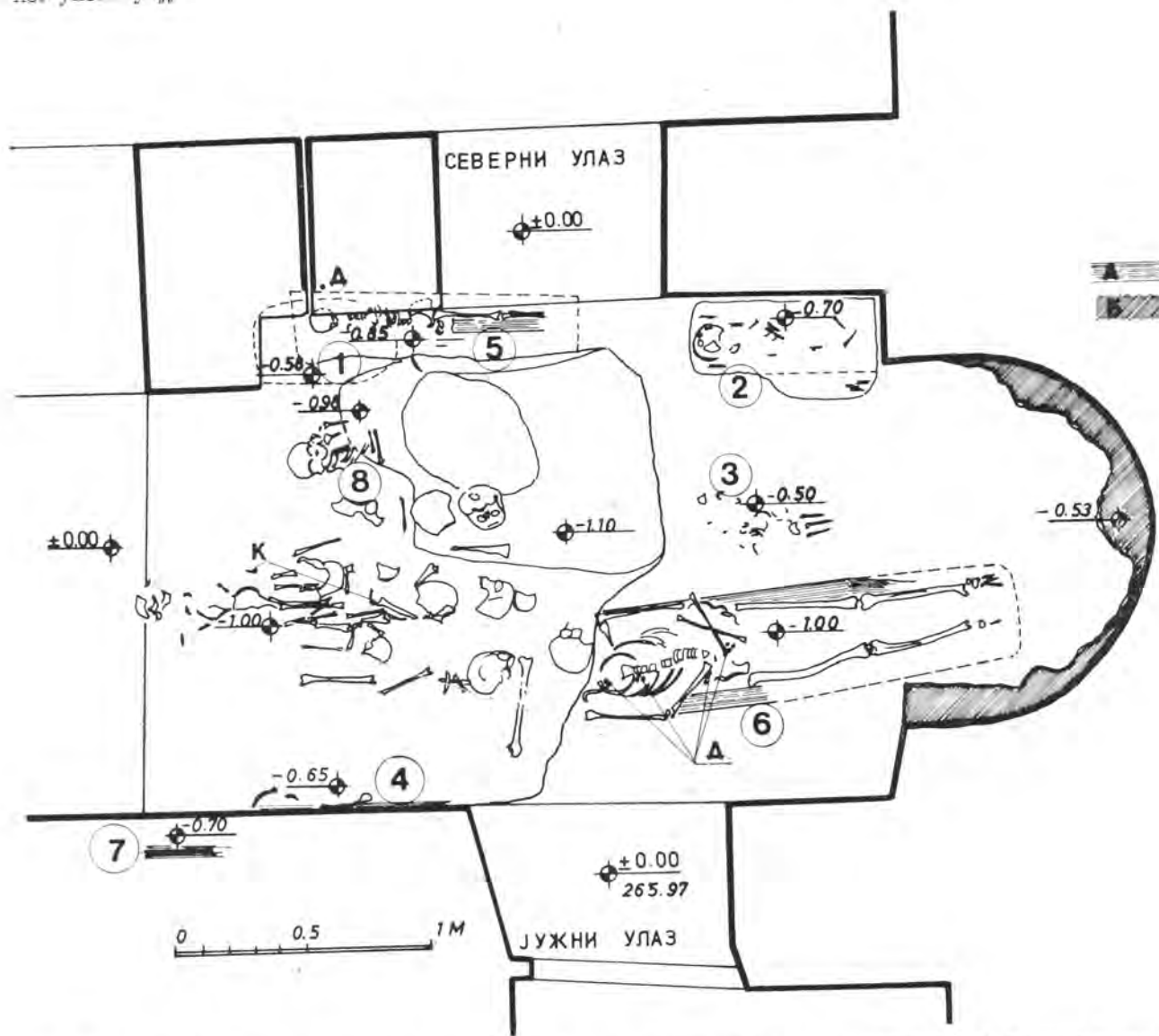
Сл. 27. — Млађи хоризонт сахрањивања, гробови 1—8 и кости из растурених гробова: А) трагови дрвеног сандука; К) гвоздени клинови; Д) бронзана дугман; И) ниво пода из X века. — Fig. 27. — Horizon récent d'ensevelissement, tombes 1—8 et groupes d'ossement provenant de tombes bouleversées; А) Vestiges d'un cercueil en bois; К) Clous en fer; Д) Doubtons de bronze; И) Niveau du sol du X e s.
