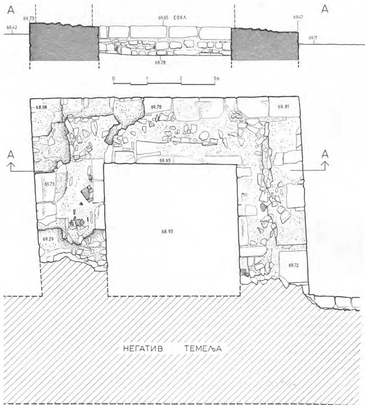
Сл. 6. — Кула I, основа са попречним пресеком (цртеж Г. Милошевић). — Fig. — 6. Tower I, foundation with cross-section (drawn by G. Milošević).
