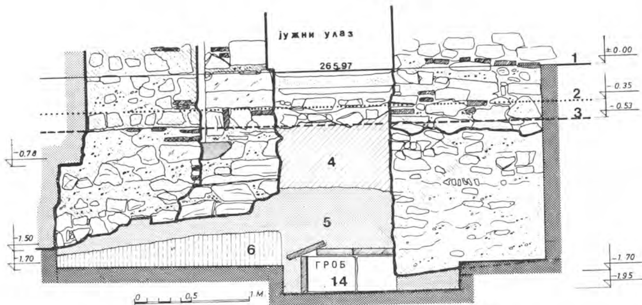
Сл. 7. — Изглед темеља јужног зида цркве у ђаконикону: 1) ниво пода из 1906. год. (садашњи под); 2) ниво пода из XI века; 3) ниво пода из X века; 4) средњевековни слој; 5) касноантички слој; 6) здравица. — Fig. 7. — Fondation du mur sud de l'église dans le diakonikon: 1) Niveau du sol de 1906 (sol actuel); 2) Niveau du sol du XI e s.; 3) Niveau du sol du X e s.; 4) Couche médiévale; 5) Couche de la basse antiquité; 6) Sol vierge.
