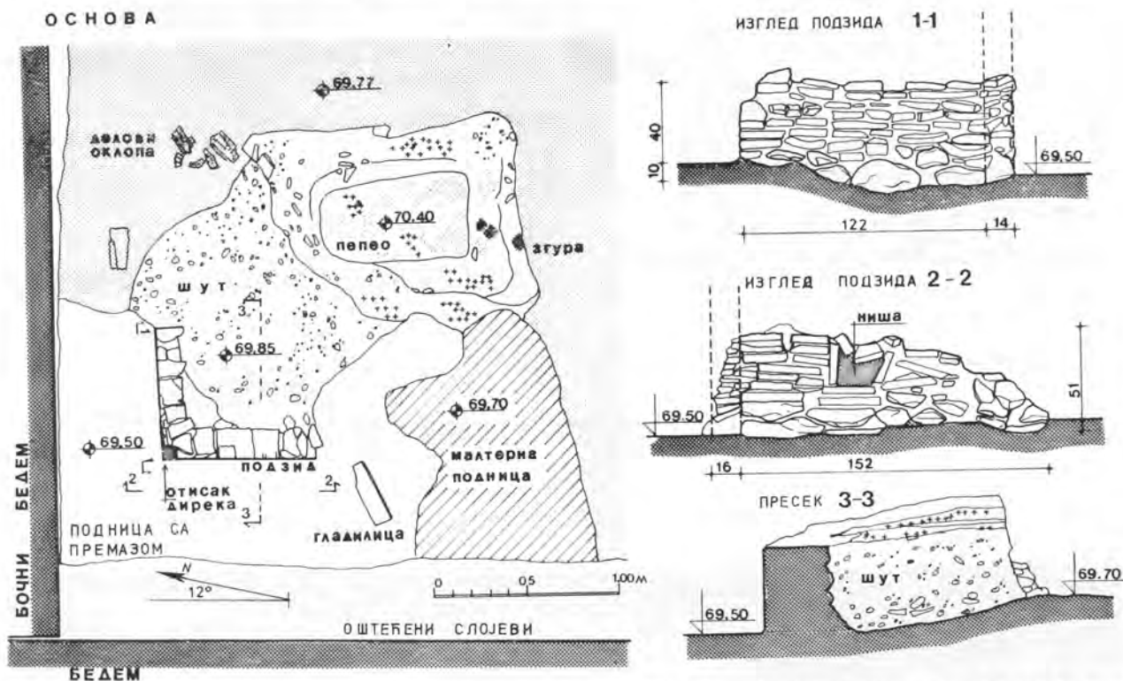
Сл. 16. — Ковачница, основа и детаљи изгледа подзида. — Fig. 16. — La forge, plan et les détails du mur de soutènement.
