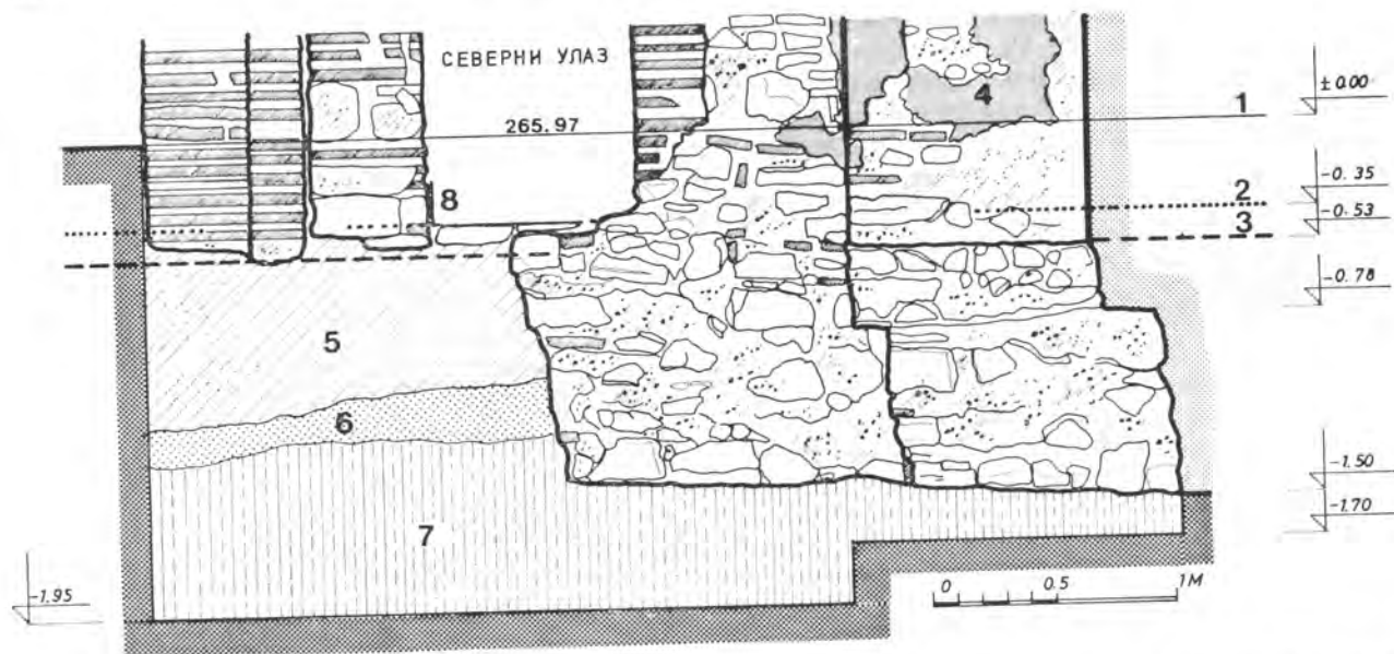
Сл. 6. — Изглед темеља северног зида цркве у ђаконикону: 1) ниво пода из 1906. год. (садашњи под); 2) ниво пода из XI века; 3) ниво пода из X века; 4) трагови најстаријег живописа (X в.); 5) средњевековни слој; 6) касноантички слој; 7) здравица; 8) трагови живописа из XI в. — Fig. 6. — Vue de la fondation du mur nord de l'église dans le diakonikon: 1) Niveau du sol de 1906 (sol actuel); 2) Niveau du sol du XI e s.; 3) Niveau du sol du X e s.; 4) Vestiges des plus anciennes fresques (X e s.); 5) Couche médiévale; 6) Couche de la basse antiquité; 7) Sol vierge; 8) Vestiges des fresques du XI e s.
