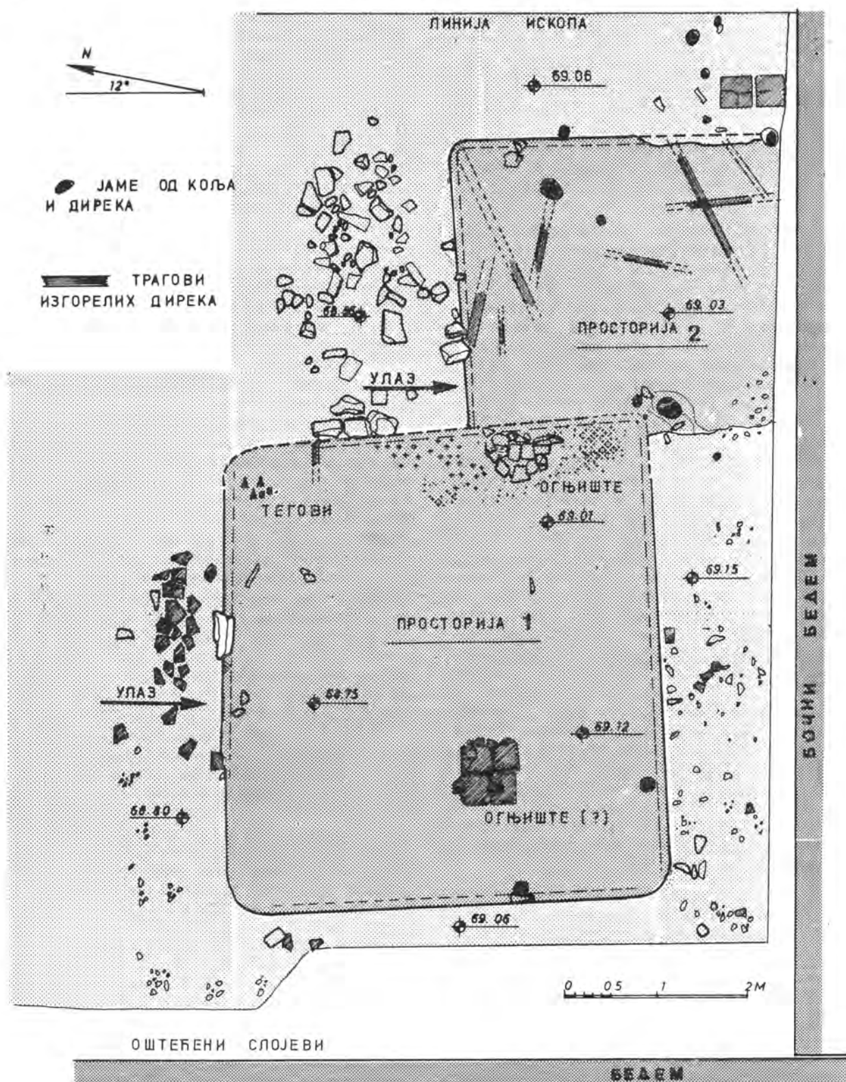
Сл. 9. — Основа куће 3. — Fig. 9. — Plan de la maison 3.
